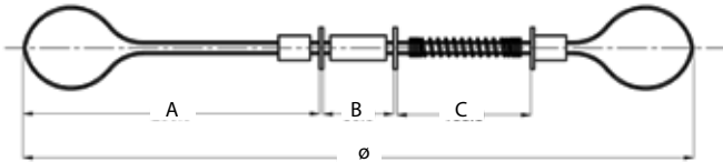
Simple Resorte
