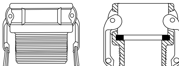
Conector B LCM Cuerpo Rosca Macho
