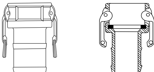
Conector C LCE Cuerpo Espiga
