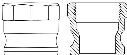
Adaptador A LNH Rosca Hembra NPT/BSP
