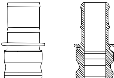
Adaptador E LNE
